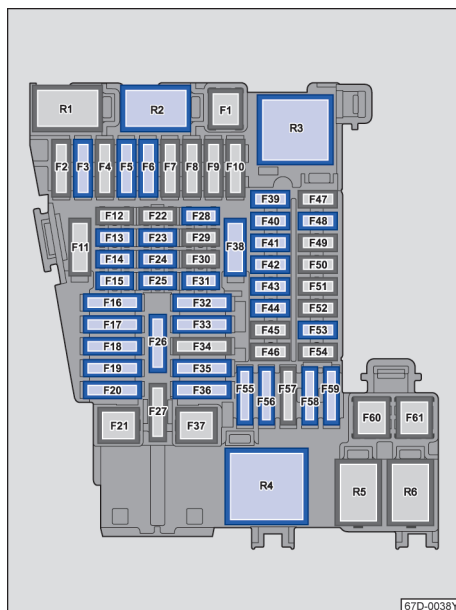
图 133 仪表板中：保险丝位置示意图
