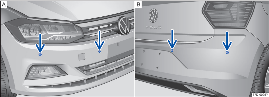
图 104 前后保险杠：驻车距离警报系统超声波传感器
