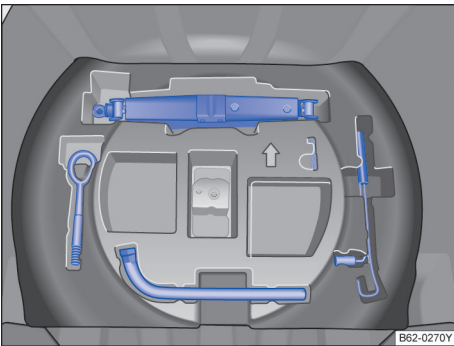
图 126 行李厢垫下的随车工具
