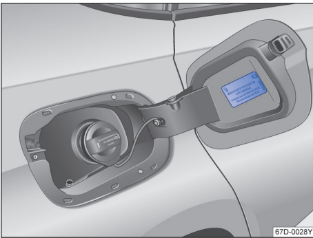
图 123 油箱加油口盖板内侧的标签
