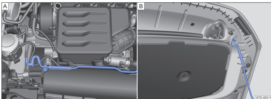
图 141 发动机舱盖支撑杆处于安放及固定位置
