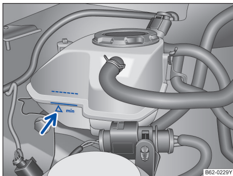
图 145 冷却液补偿容器上的液位标记
