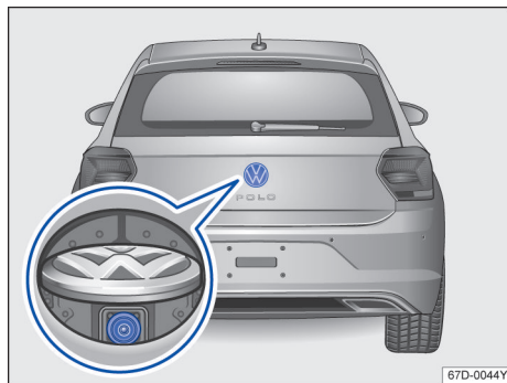
图 108 车辆行李厢盖内：倒车摄像头的安装位置
