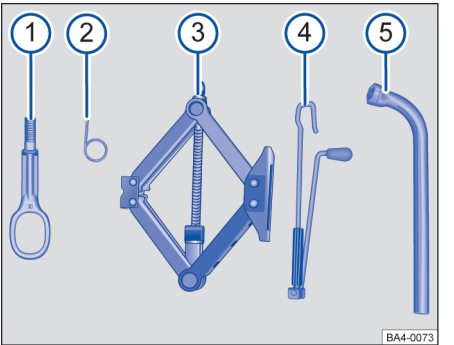
图 127 随车工具的组件
