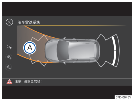
图 107 泊车雷达系统显示屏：施加转向时汽车行驶路径显示模式
